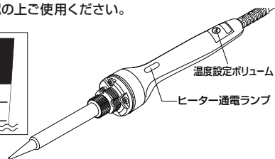
温度設定ボリューム ラベル
